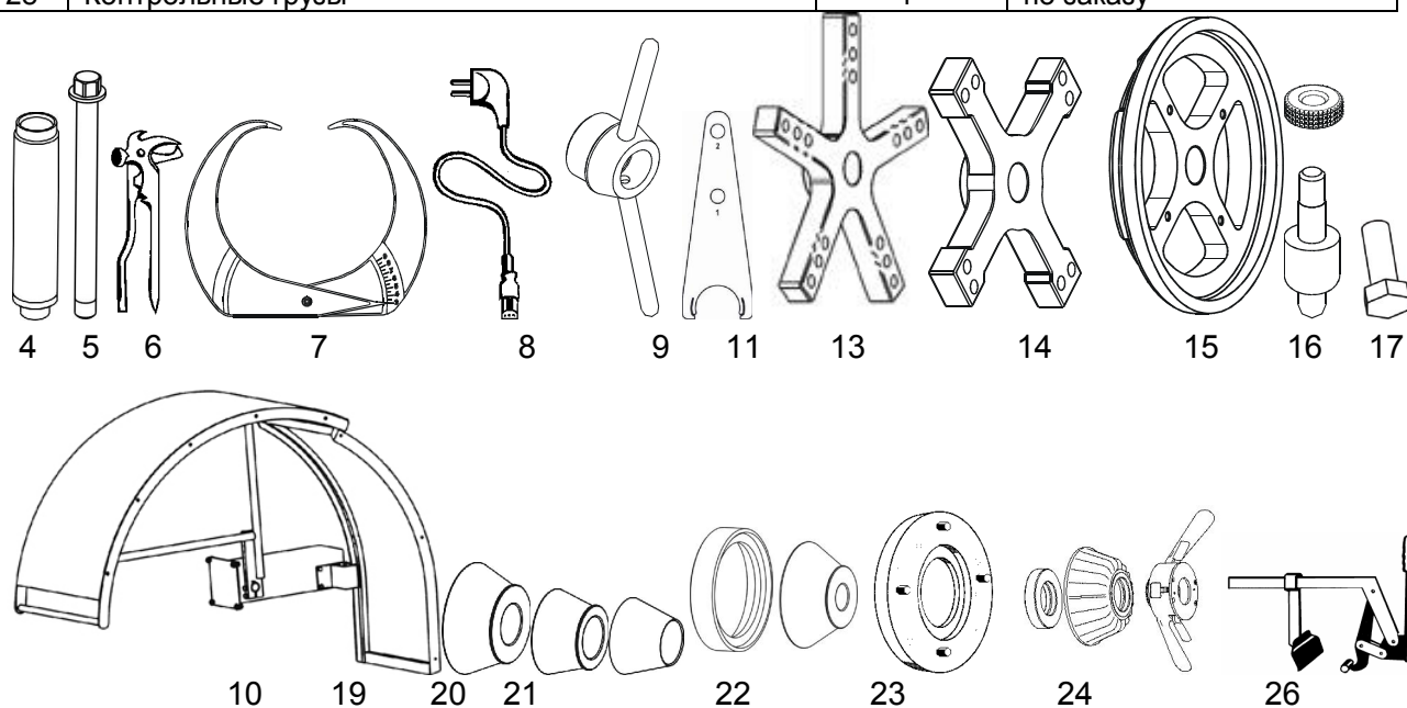
Рисунок 3.1 – Поставляемые принадлежности
